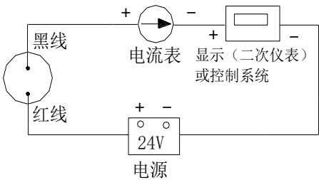
二线制电流 4mA~20mA 叠加 HART 输出接线图
