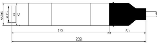
投入式隔爆液位变送器尺寸
