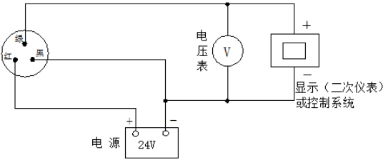
RS485 网络型接线图
