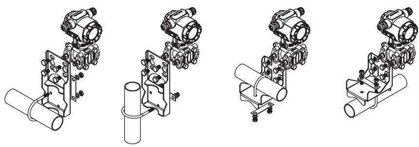
使用水平支架安装图
