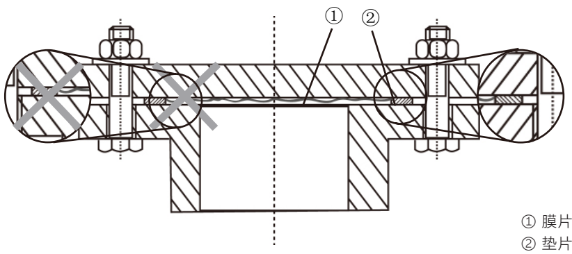
图 19：法兰或膜盒安装方式
