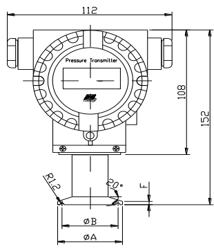
WP 卫生型压力变送器卡箍式快接法兰尺寸
