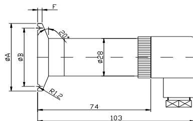
WH 卫生型压力变送器卡箍式安装尺寸
