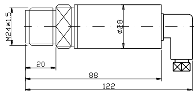
WH 卫生型压力变送器螺纹安装尺寸
