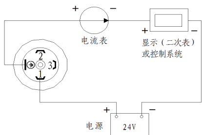
二线制电流 4mA~20mA 输出接线图(JYB-KB-WPA***)
