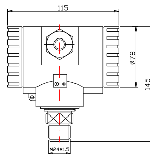
WP 卫生型压力变送器螺纹安装尺寸
