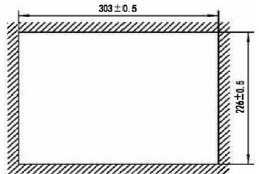
开孔尺寸
