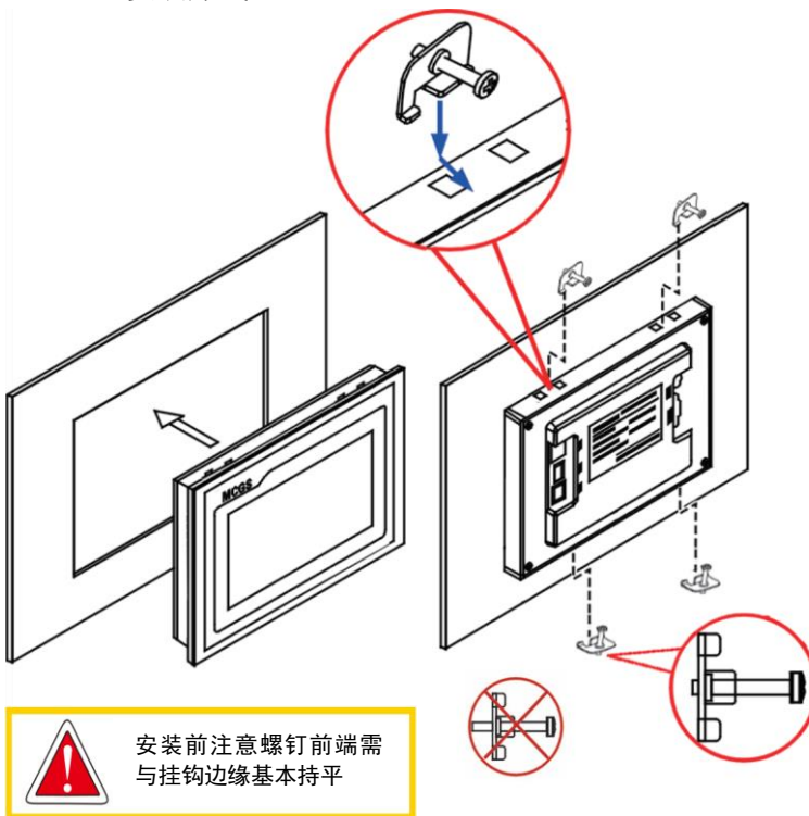
挂钩安装
