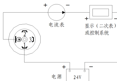
三线制 0V~5V 电压输出接线图(JYB-KO-HV*)
