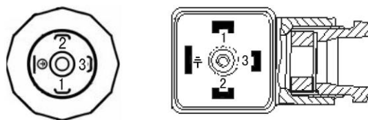
二线制 4mA~20mA 电流输出接线图(JYB-KO-HA*)
