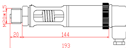
高温型压力变送器螺纹安装外形
