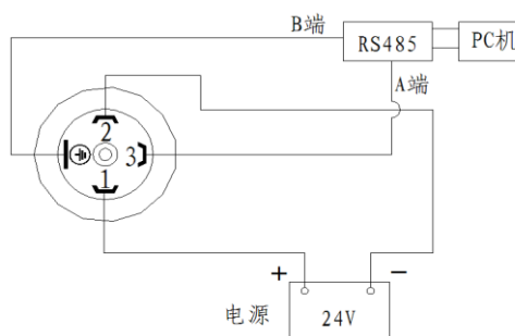
RS-485 网络输出接线图(JYB-KO-HW1*)
