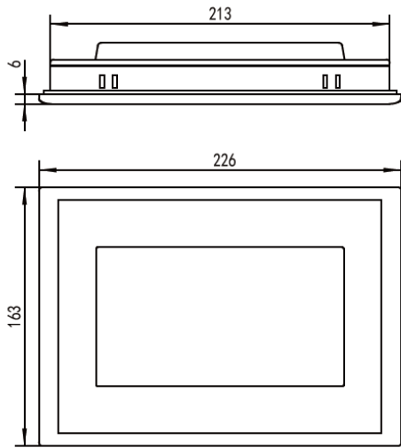
外形尺寸
