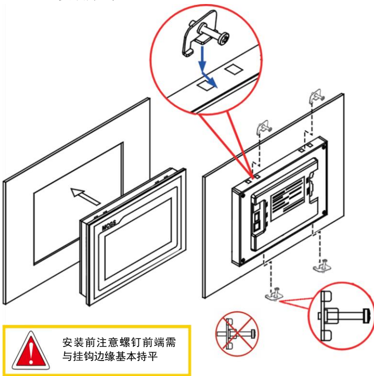
挂钩安装
