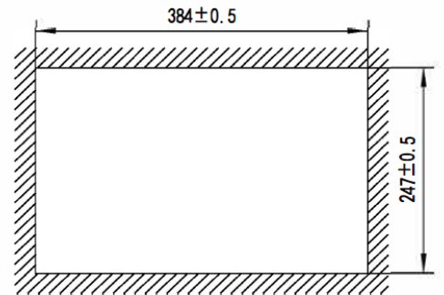
开孔尺寸
