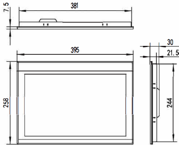
外形尺寸
