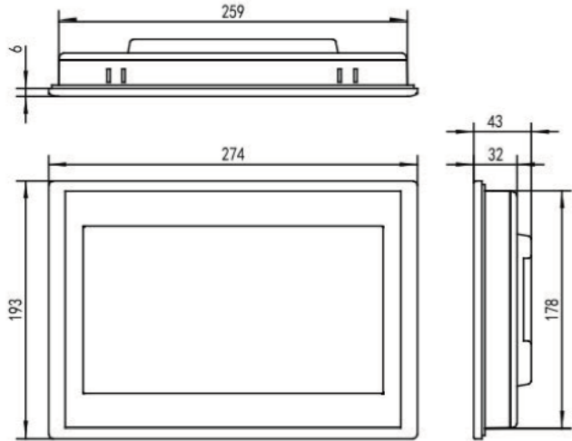
外形尺寸
