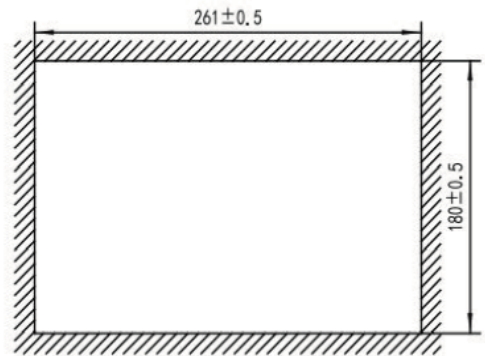
开孔尺寸
